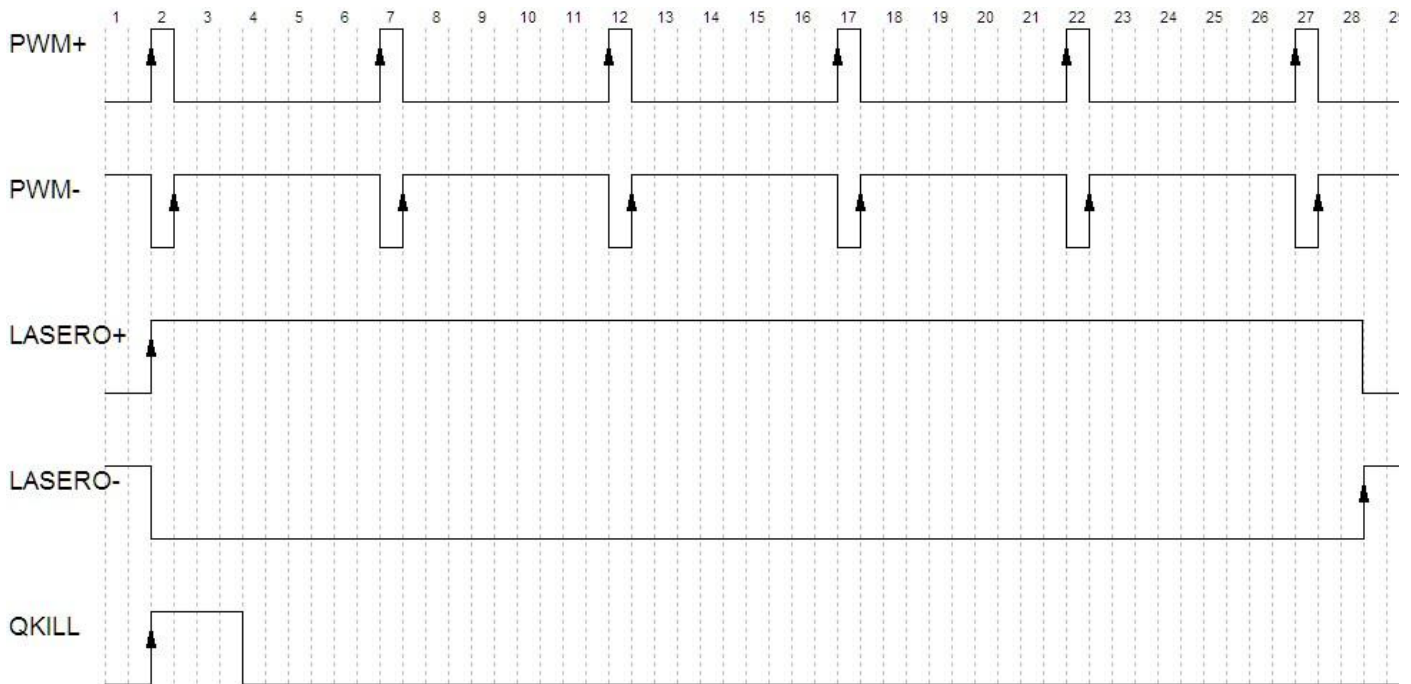
YAG 激光器波形图
