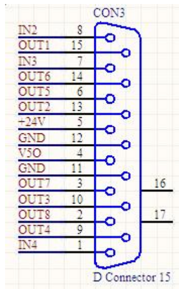
图 5 拓展 IO 接口对应图
