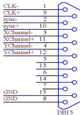
图 3 实际振镜接口对应图
