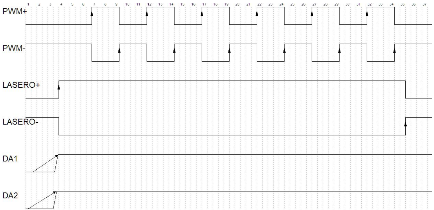
模拟激光器波形图
