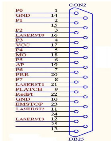
图 4 激光接口对应图
